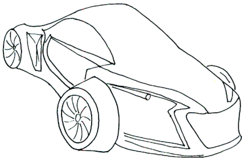
AUTO BUDOUCNOSTI
